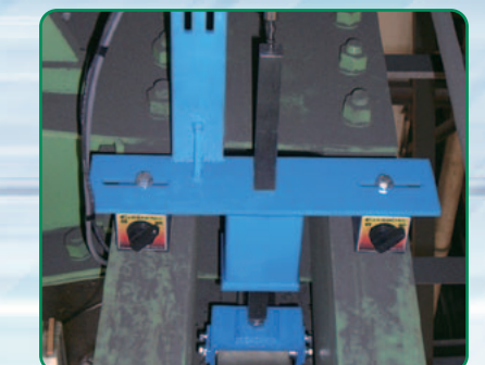
レールレベル測定装置外観
