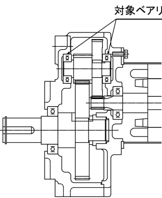
図 1. 対象ベアリング位置 (0.4kW～2.2kW)
