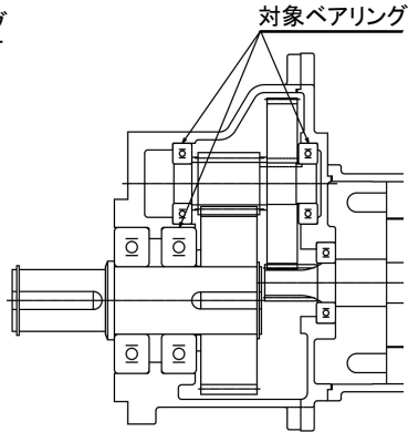
図 2. 対象ベアリング位置 (3.7kW)
