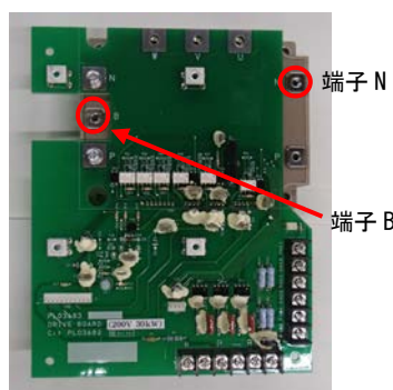
図 2. 変更品 (03G5A0、03G5A1)
