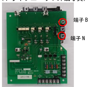
図 1. 従来品 (03G510)
