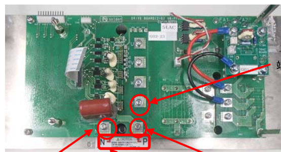
端子 N 注意喚起シール 端子 P 端子 B 図 2. 切替品
