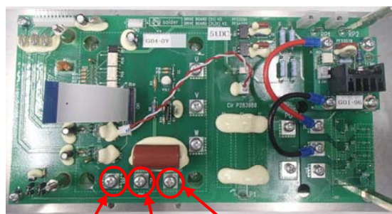
端子 B 端子 P 端子 N 図 1. 従来品
