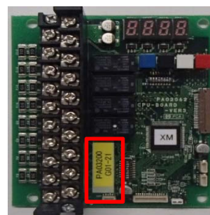
図2 クレーンリモート非対応基板
