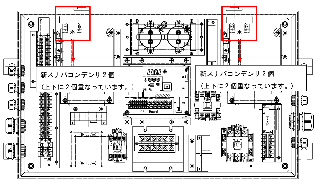
新 200V 級 US-7.5kW(5t) の制御箱
