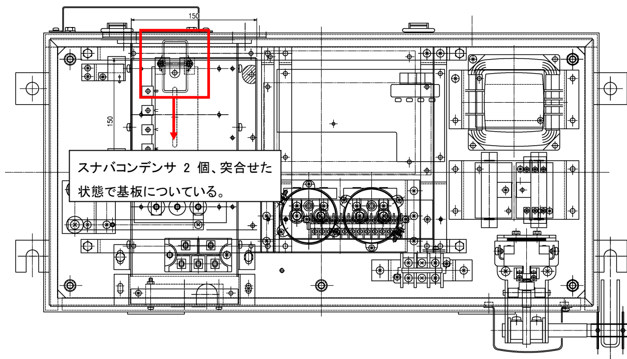
新 400V 級 U2-12kW(10t) 制御箱
