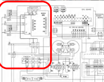
<新制御箱>
