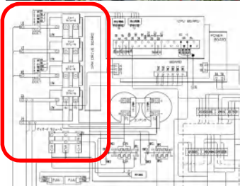
<旧制御箱>
