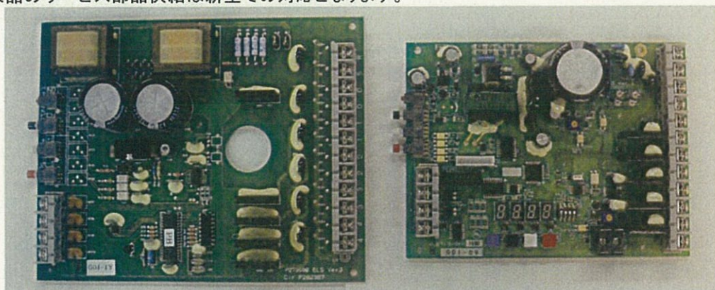
旧 ELS 基板(左)及び新 ELS 基板(右)外観写真
