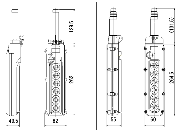
変更前（春日電機製 6点押釦）
