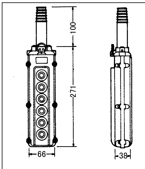
変更前 (新晃電機製 6点押釦)
