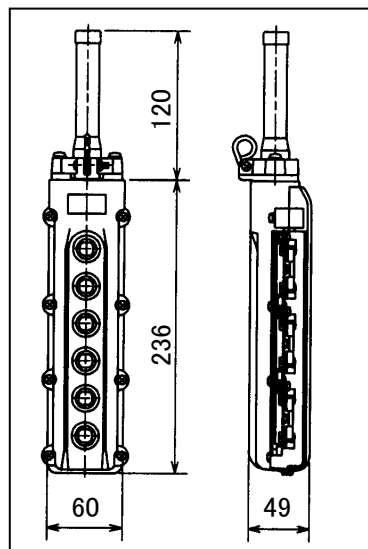
変更後 (春日電機製 6点押釦)
