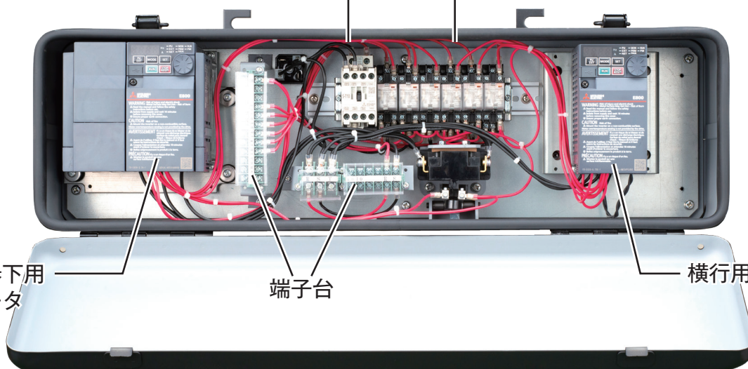
制御箱内機器配置(全機種共通) ブレーキ用接触器 リレー
